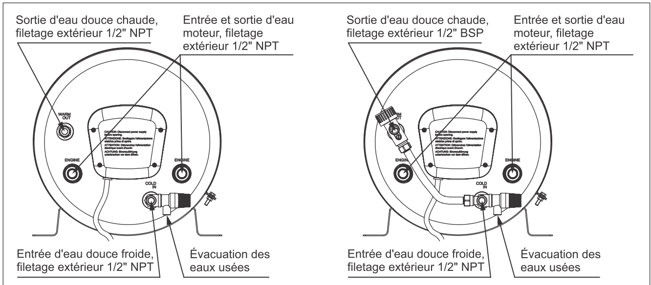
Fig. 4 S'il vous plaît notez: Les raccords de manches par droites 1/2 BSP correspondent également au 1/2 " filetage extérieur de type NPT.
