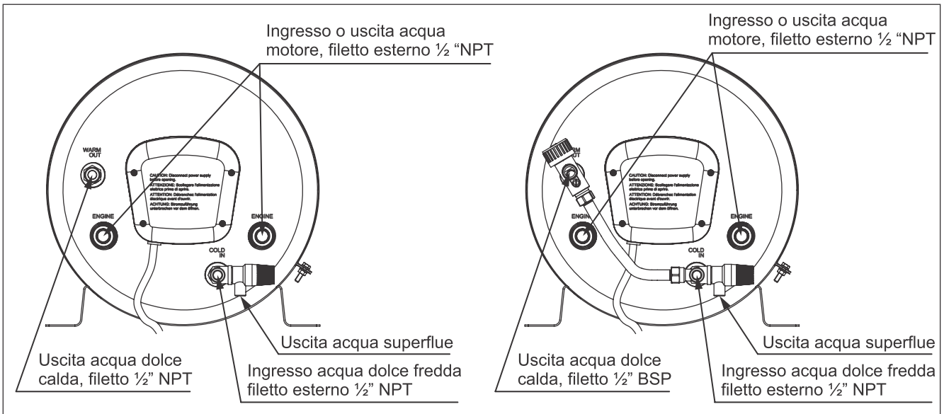
Fig. 4 Nota: Raccordi per tubi flessibili con filetti dritti 1/2" BSP si adatta anche a 1/2" NPT filetto esterno.
