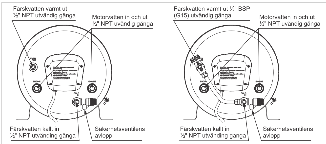
Fig. 4 Observera: Slangnipplor med rak 1/2" BSP gänga passar även till 1/2" NPT utvändig gänga.
